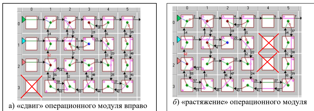
Рис. 2. Преобразования топологии микропрограммных модулей на ячейках ассоциативной памяти
