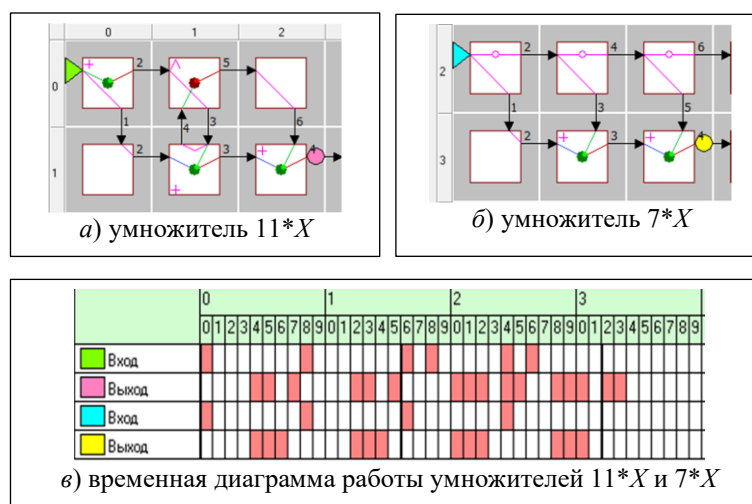
Рис. 1. Топологические схемы и временная диаграмма работы PD -ассоциативных умножителей
