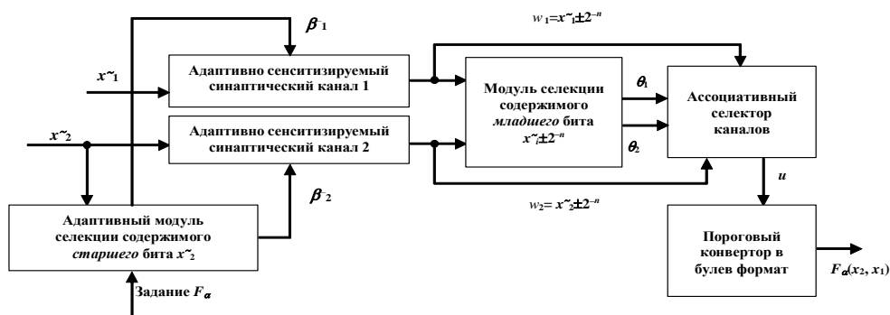
Рис. 4. Функциональная схема работы адаптивно сенситизируемых постсинаптических каналов
